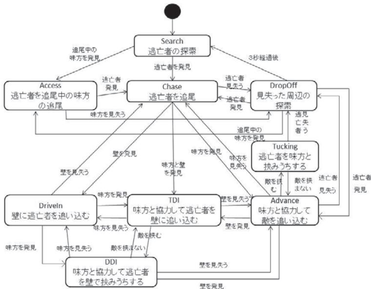
図8 協調AIのFSM図
