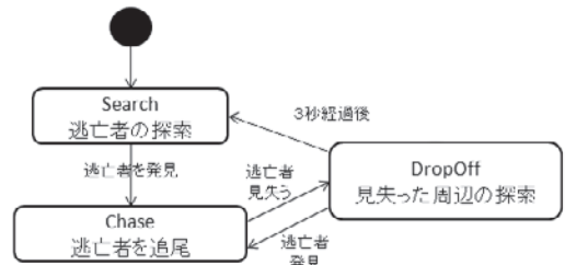
図7 単純AIのFSM図
